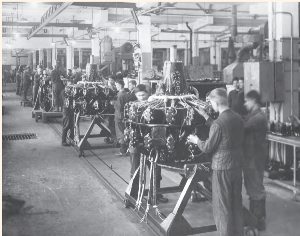
Сборочный цех завода им. Свердлова
